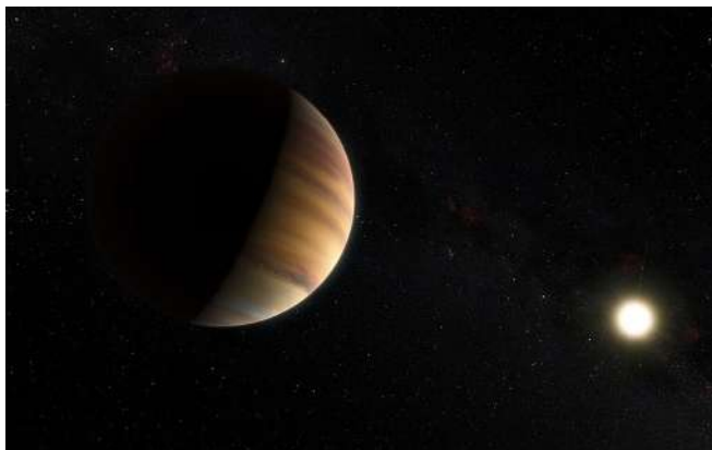
Slika 2 – Umjetnički prikaz objekta 51 Pegasi b, prvog ekstrasolarnog planeta otkrivenog 1995. godine (izvor: ESO/M. Kornmesser/Nick Risinger)
